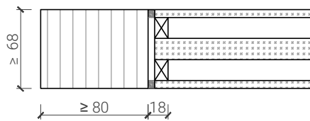
Plano-Verglasung
