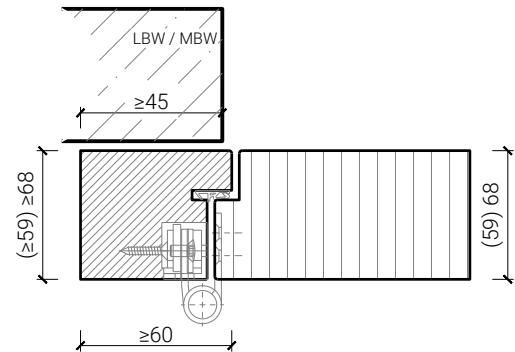
Blockrahmen 59 / 68 mm, Türe stumpf
