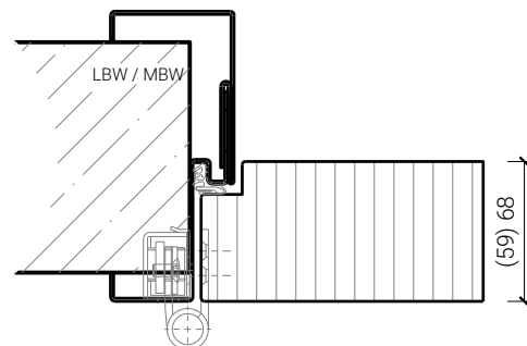
Zweiteilige Stahlumfassungszarge, Türe stumpf
