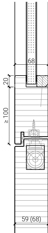
Türe / Oberteil verglast* integrierter Türschliesser*
